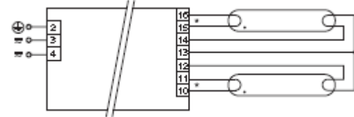
Wiring 7
