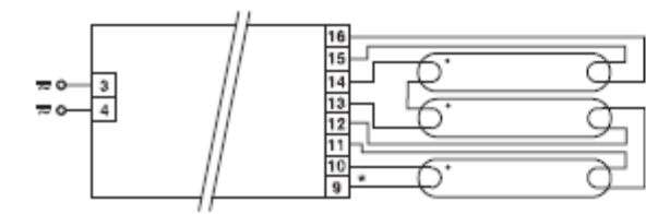
Wiring 5
