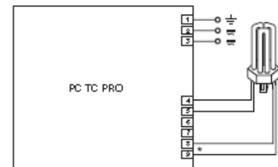
Wiring 13 & 14
