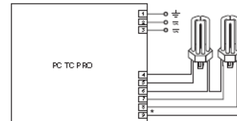
Wiring 12
