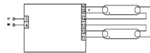
Wiring 3
