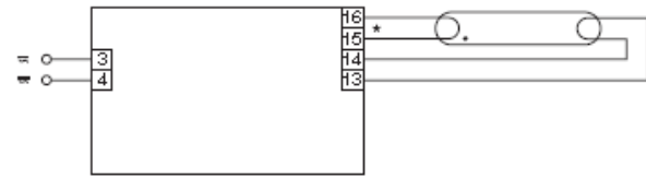
Wiring 1
