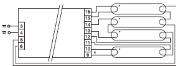
Wiring 6
