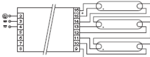
Wiring 9 & 10
