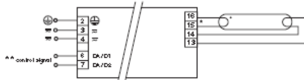
Wiring 13 & 14
