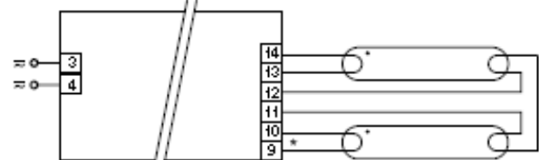
Wiring 4
