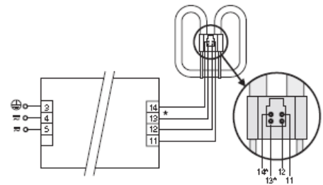
Wiring 8
